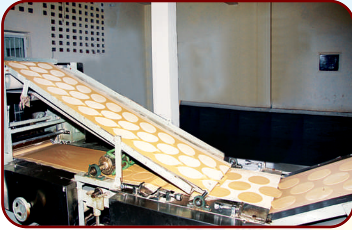
संक्रामक रोगों से बचाव हेतु चपाती बनाने की स्वचालित मशीन
